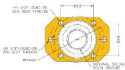
SAE B Flange
