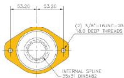
SAE A Flange
