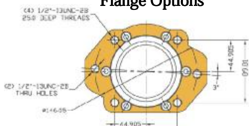
SAE B Flange
