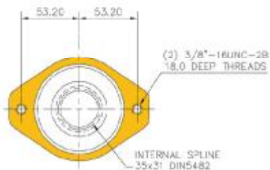
SAE A Flange
